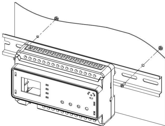
2) 产品安装尺寸示意图:
