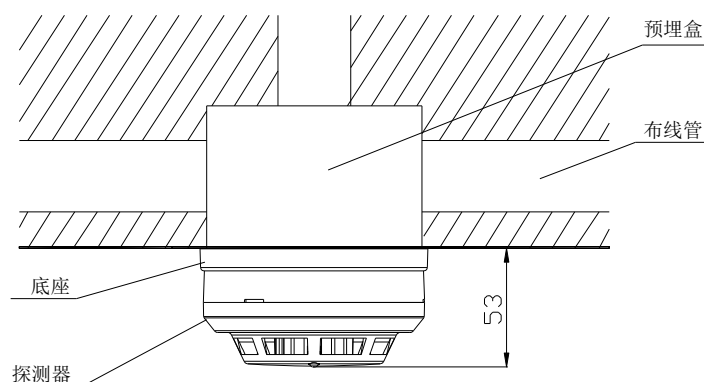
图 2 探测器安装示意图
