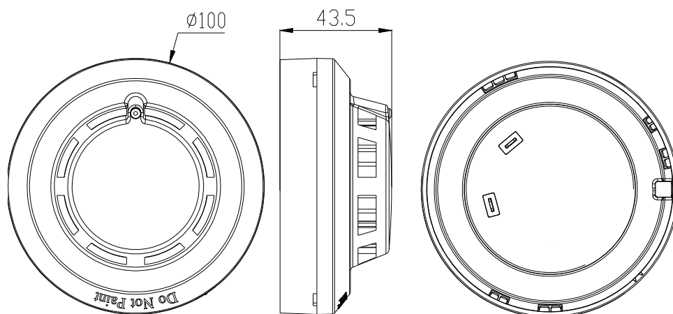
图 1 探测器外形示意图
