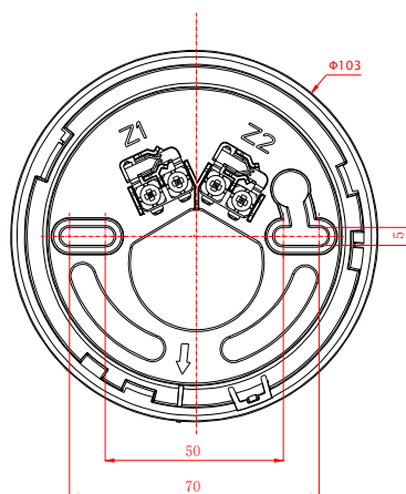
图3 探测器底座外形示意图
